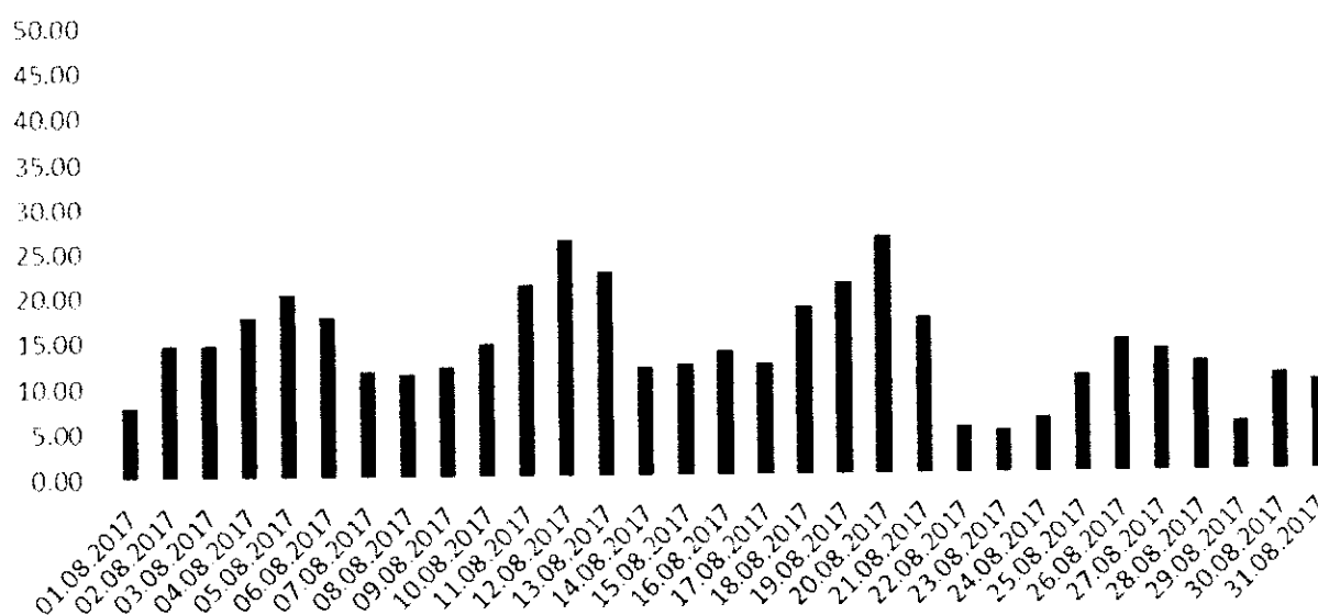
PM10 gravimetric \mu\text{g}/\text{m}^3 - Perioada 01 august - 31 august 2017-Date validate Valoarea maximă zilnică 50 \mu\text{g}/\text{mc}
